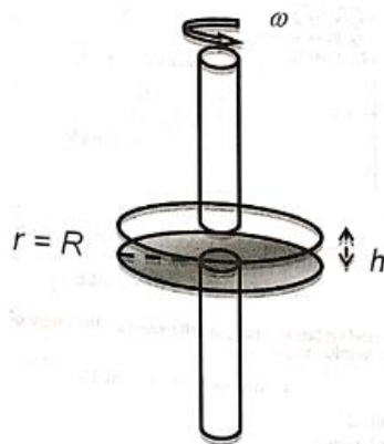
Gambar 7. Rheometer rotasional lempeng paralel
