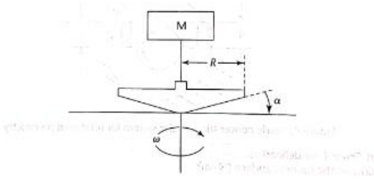
Gambar 5. Rheometer rotasional kerucut dan lempeng dengan kerucut berputar
